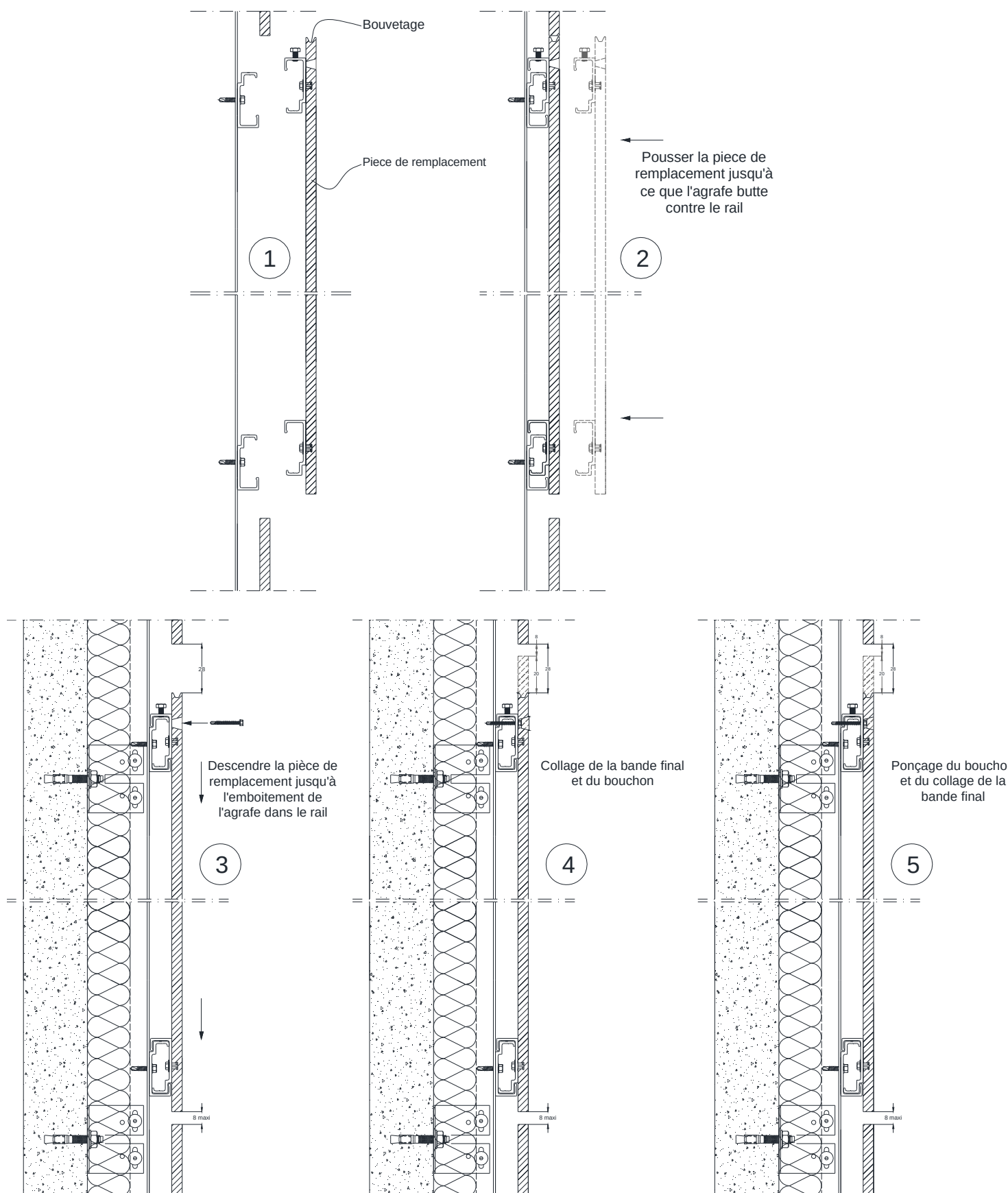
Figure 52.1 - Remplacement d'un élément
