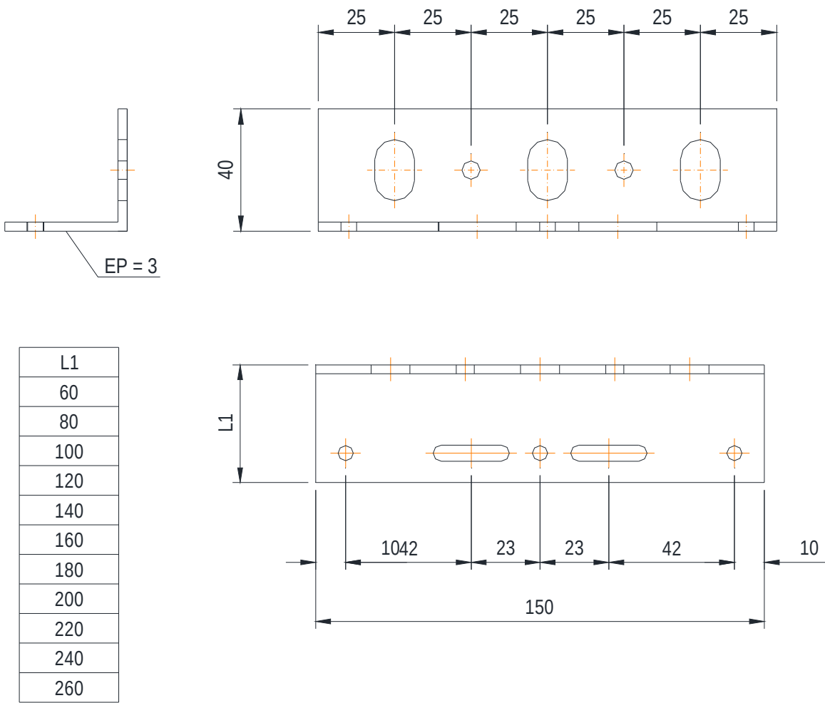
Figure 45 - Equerre LR 150 pour plan incliné
