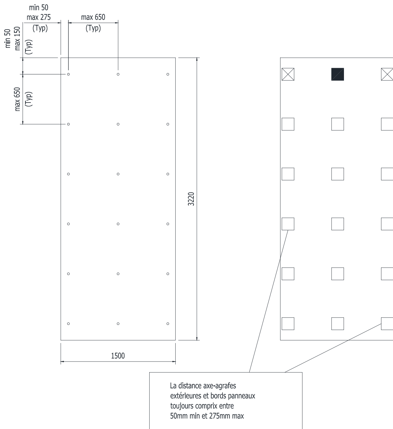
Figure B3- Schéma de panneau et positionnement des inserts
