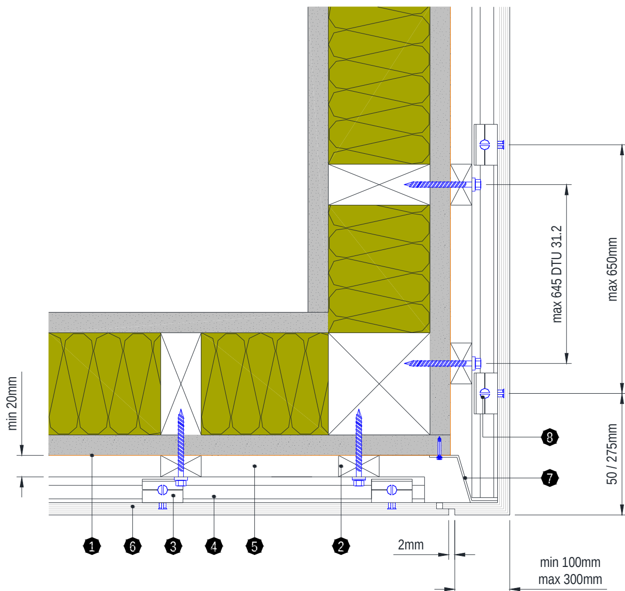
Figure 42.2 - Coupe angle sortant (panneaux monobloc à feuillure)
