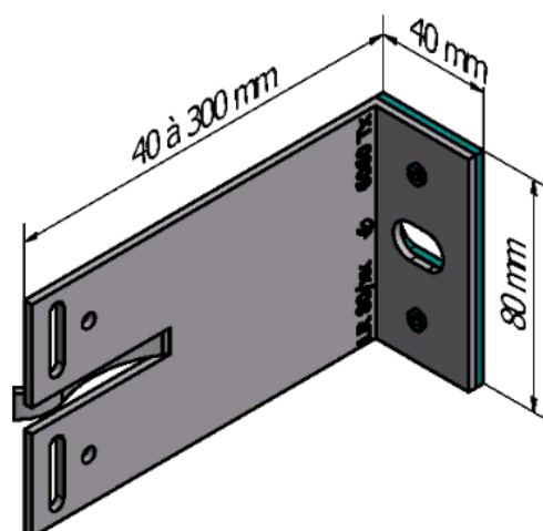
Figure 5.3 - Patte-équerres MFT-MFI du système HILTI
