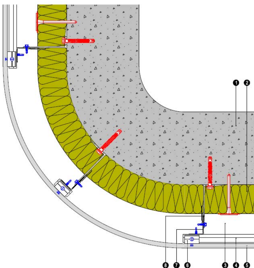
Figure 29.5 - Angle de bâtiment cintré intérieur (rayon de courbure selon §2.2.2).
