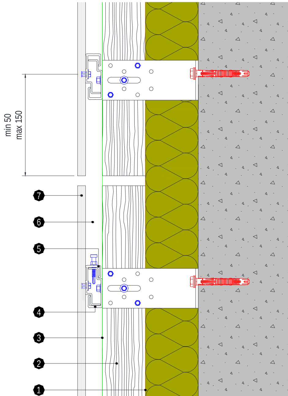
Figure 38.1 – Fractionnement de l'ossature : Chevrons de longueur \leq 5,40\text{m}
