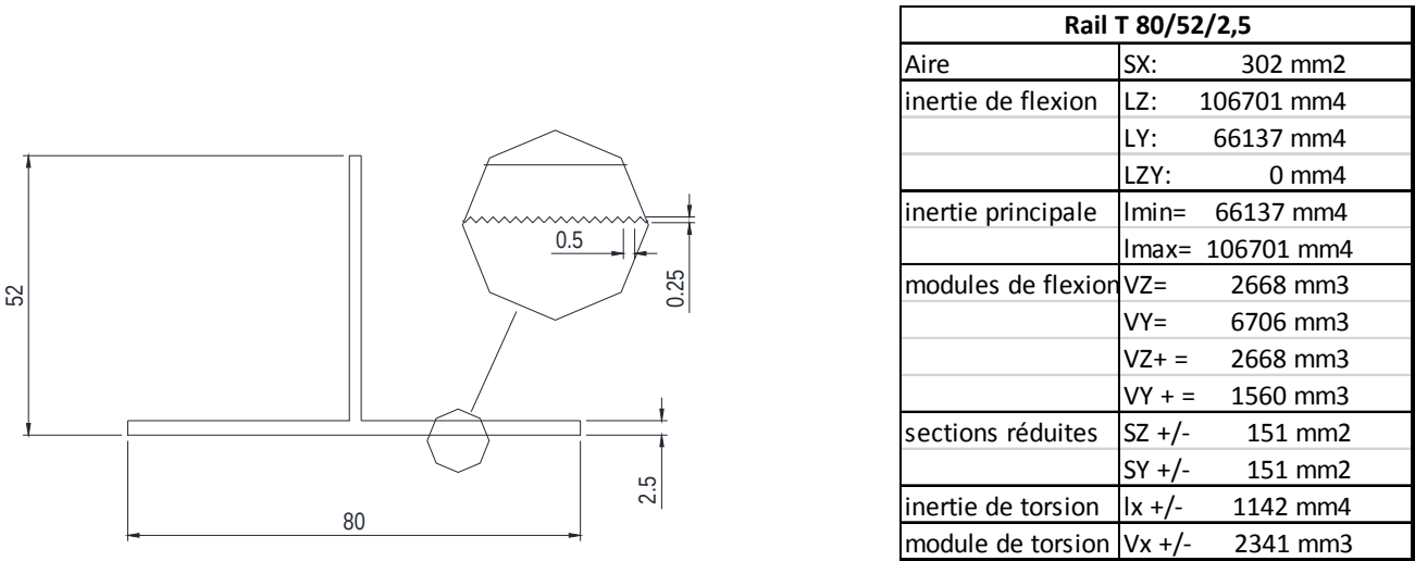
Figure 44 - Rail T 80/52 pour plan incliné
