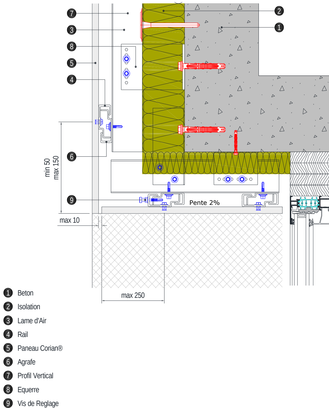
Figure 23.3 - Linteau avec habillage en panneaux DuPont Corian® EC – Solution 2
