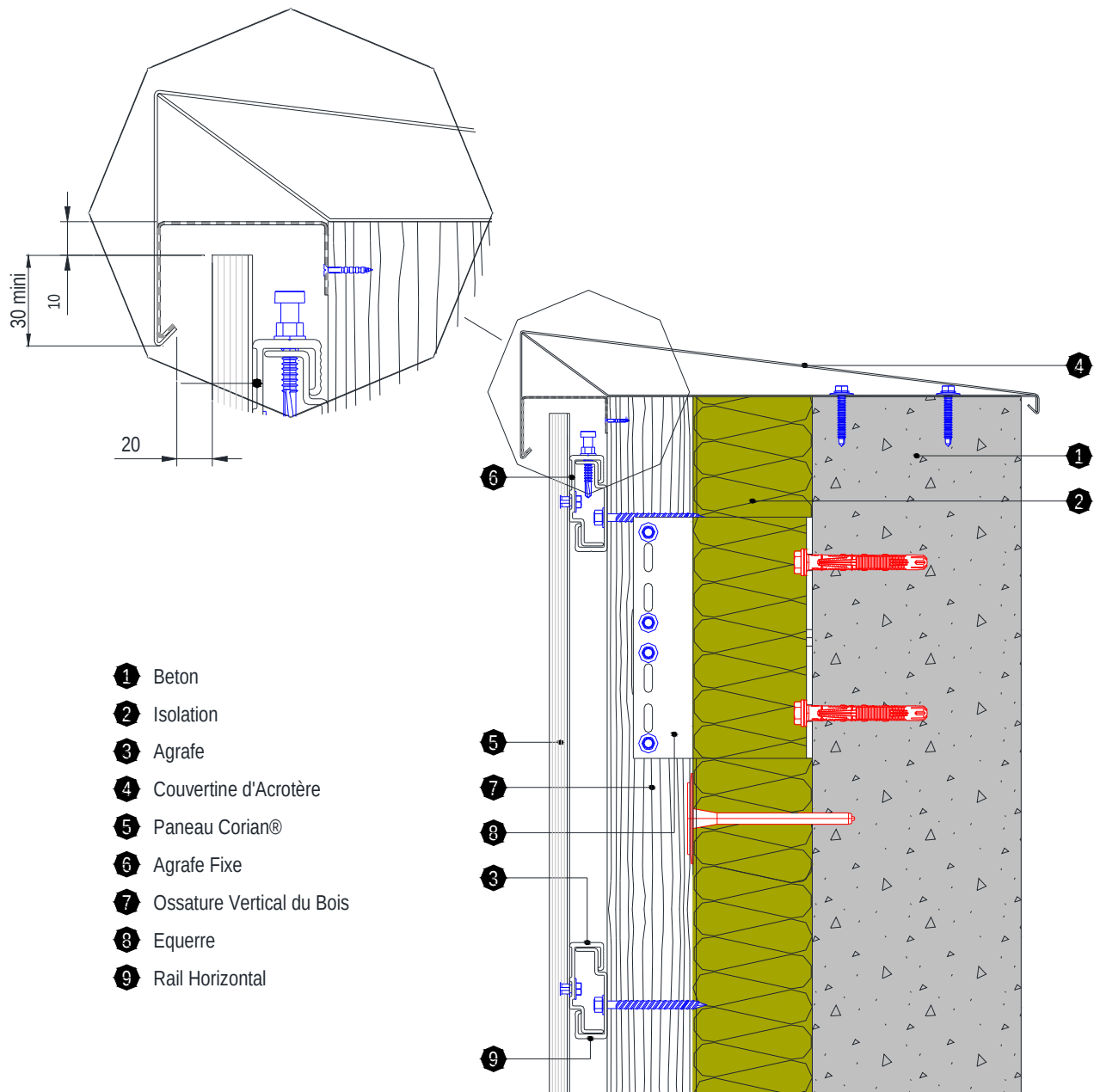
Figure 34 – Acrotère
