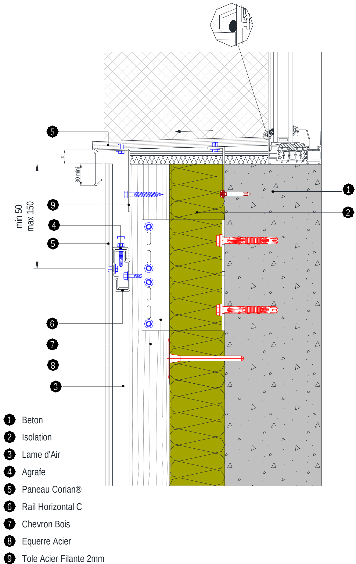
Figure 36.1 - Appui fenêtre Corian® sur ossature bois
