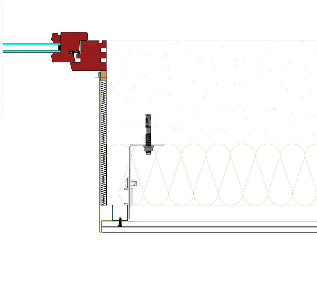
Figure 11 – Coupe sur encadrement de baie en acier
