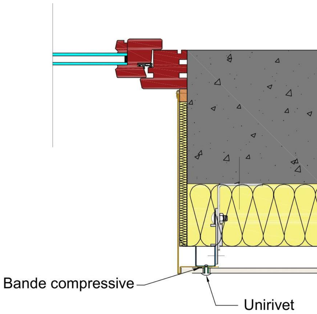
Figure 2 - Coupe sur encadrement de baie en acier
