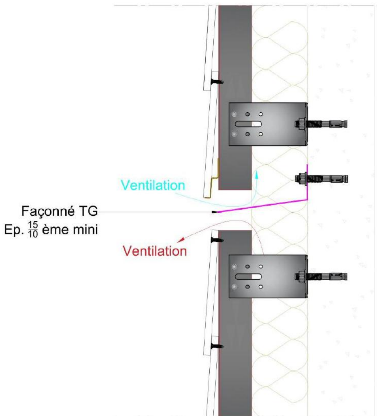
Figure 10 – Détail de recouplement avec recouplement
