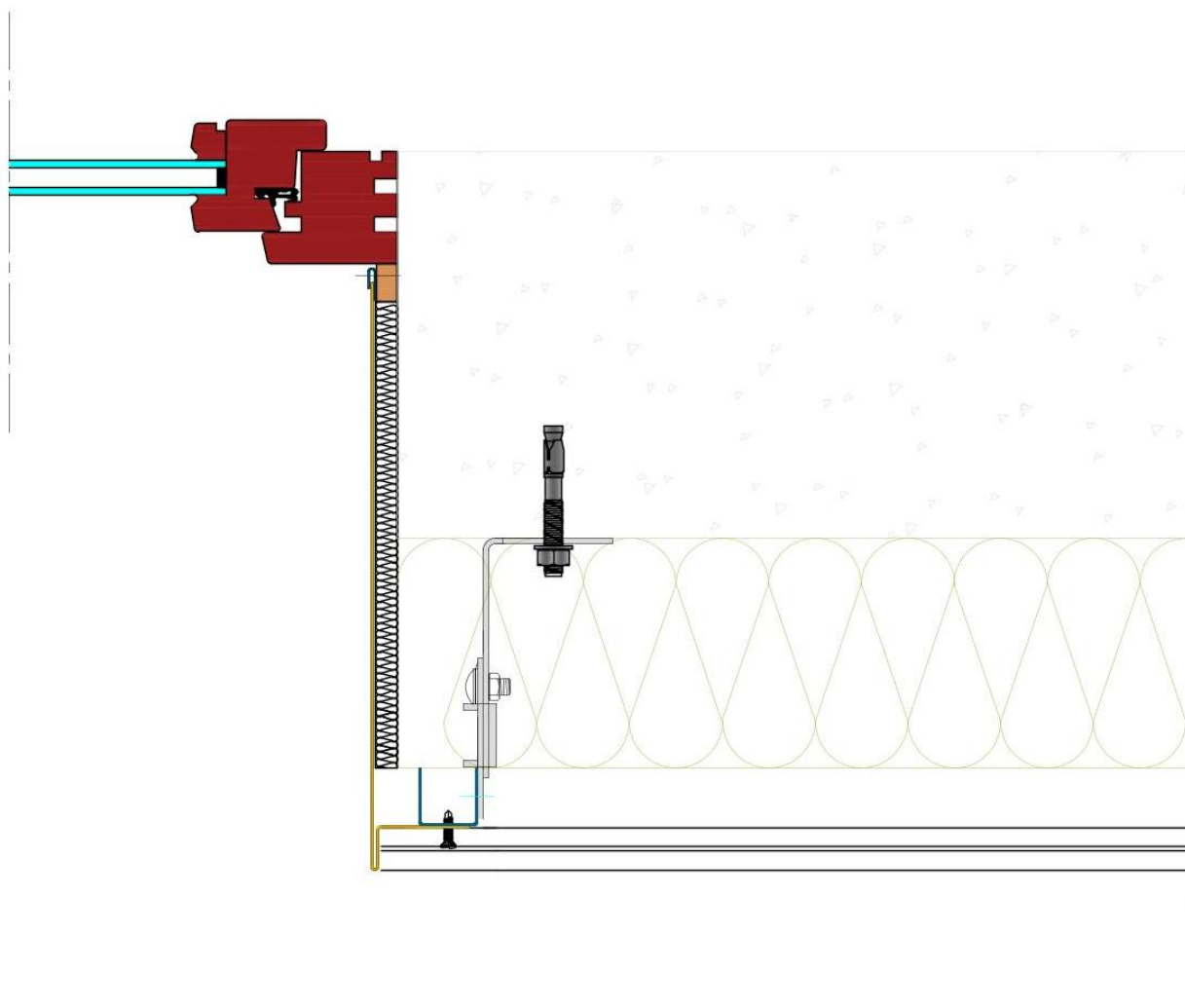
Figure 12 - Encadrement de baie en retour de parement
